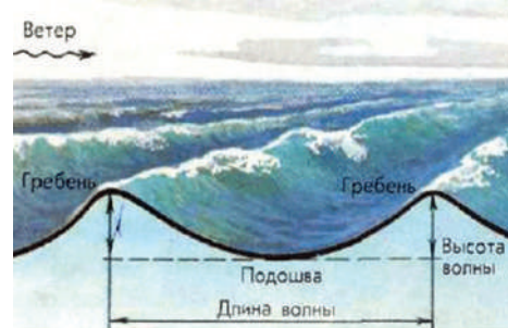
Ветровая волна
